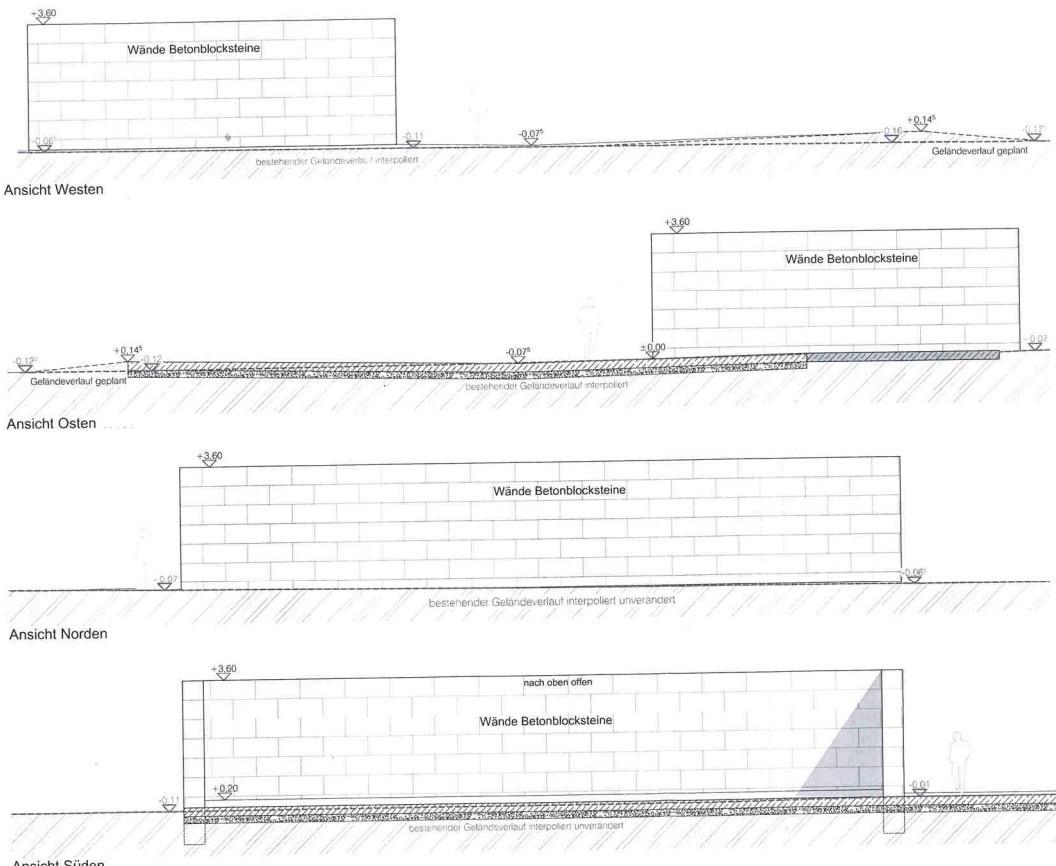
Auszug Ansichten zum Bauantrag
