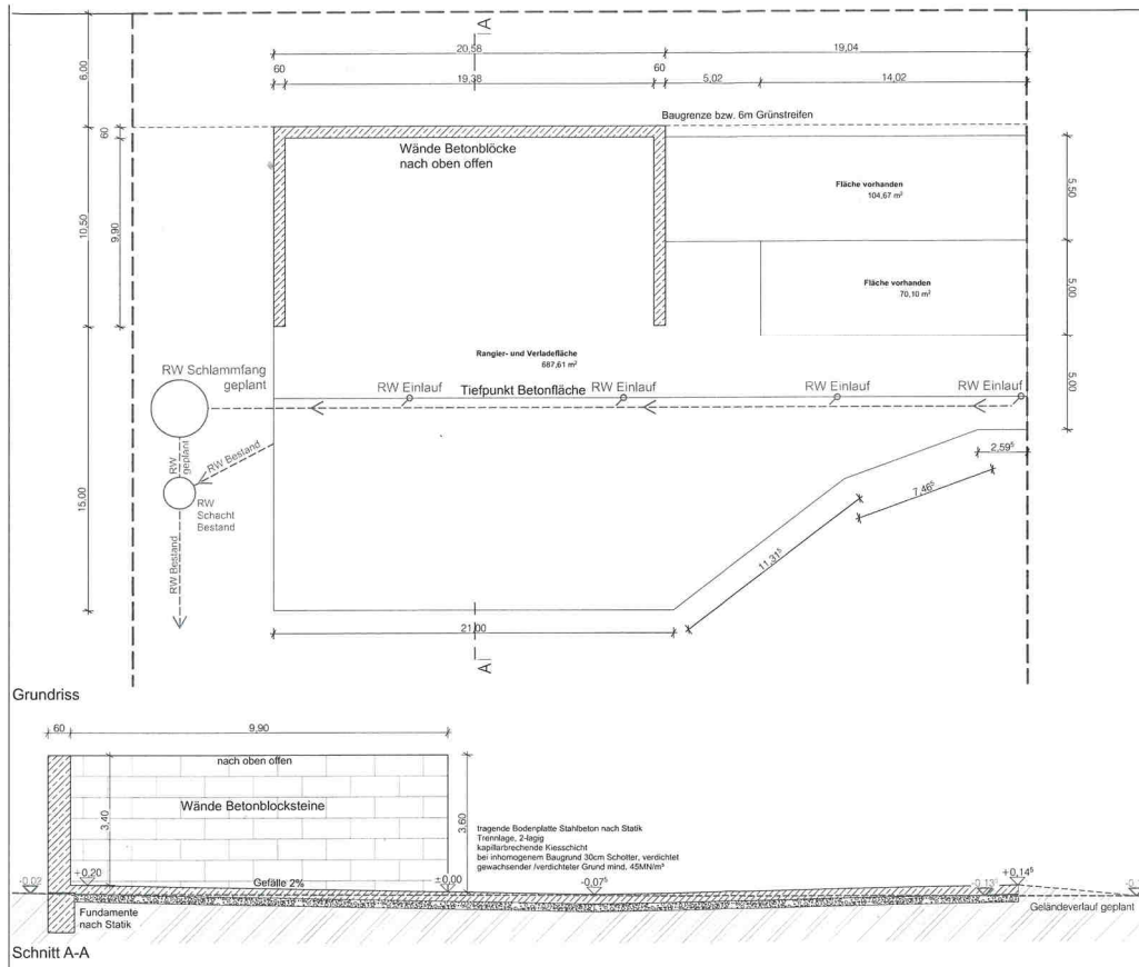
Auszug Grundriss und Schnitt zum Bauantrag
