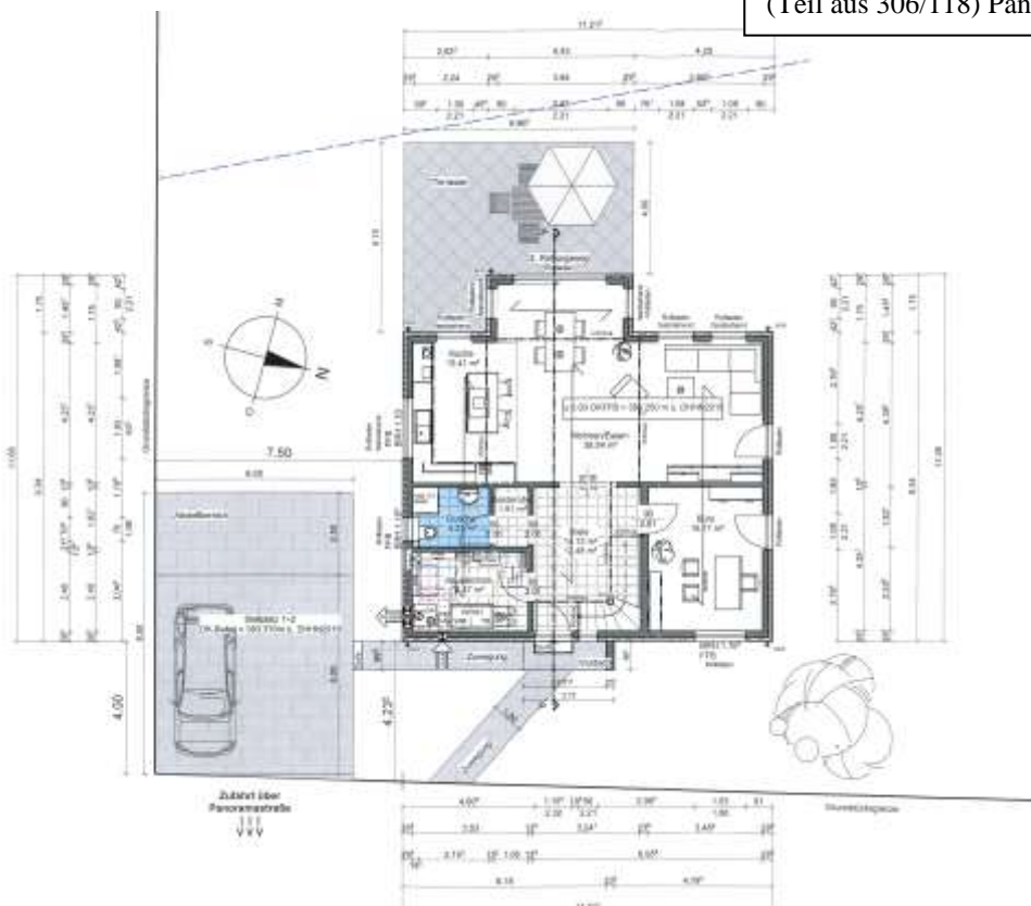
Auszug Grundriss Erdgeschoss zum Bauantrag
