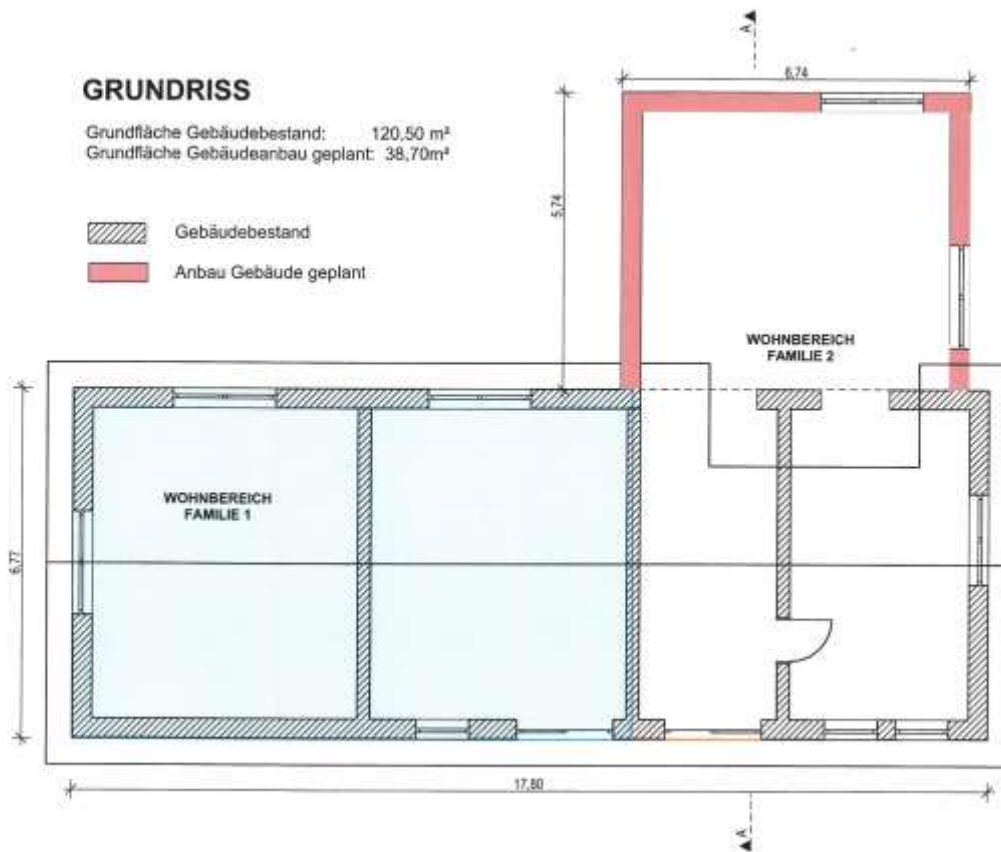
Auszug Grundriss-Schema zum Bauantrag
