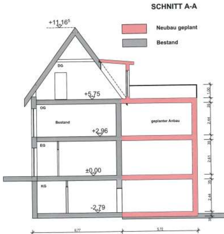
Auszug Schnitt-Schema zum Bauantrag
