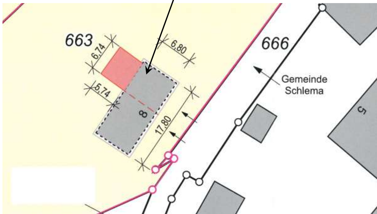
Auszug Lageplan zum Bauantrag
