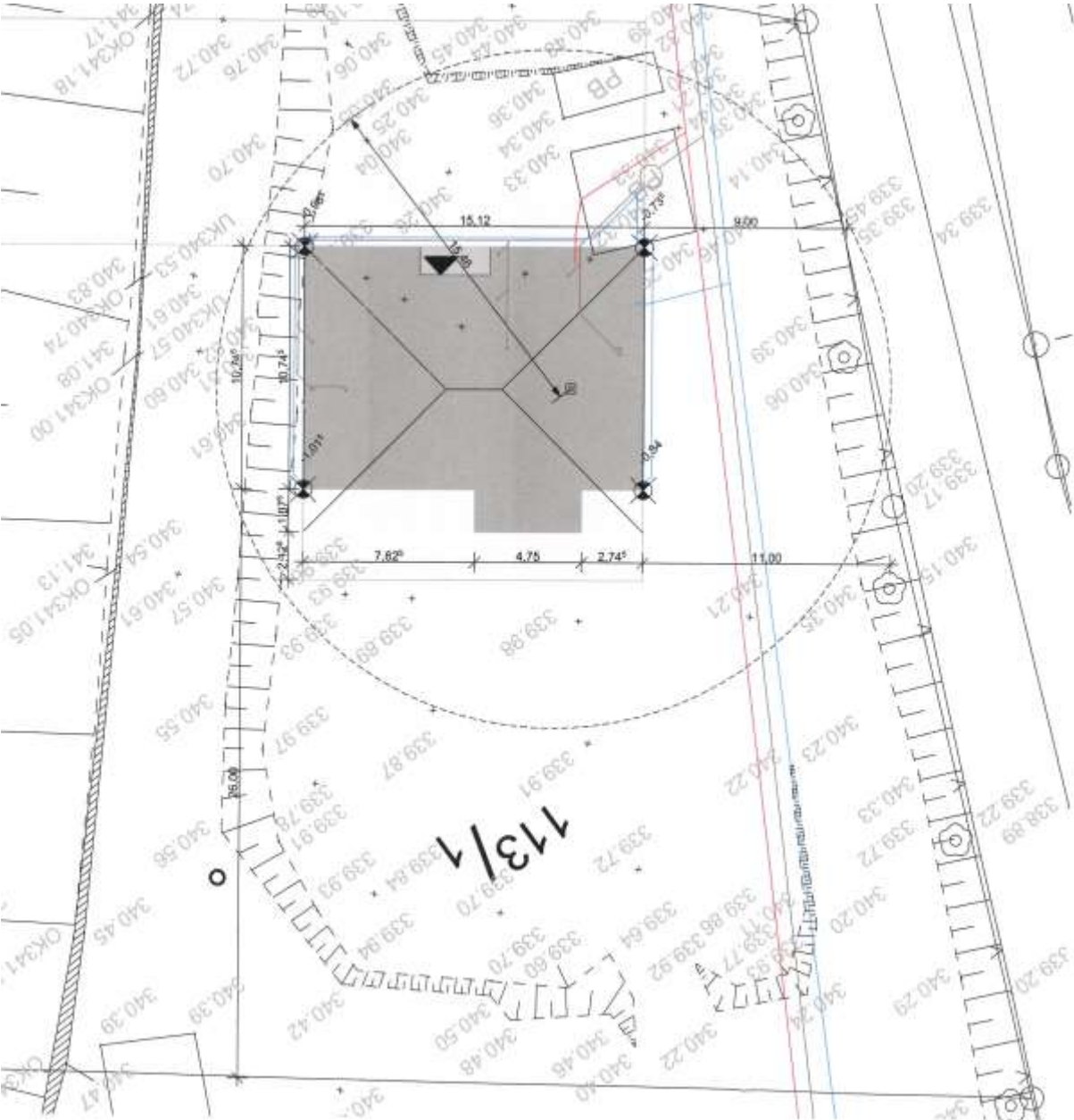
AuszugLageplan zum Bauantrag
